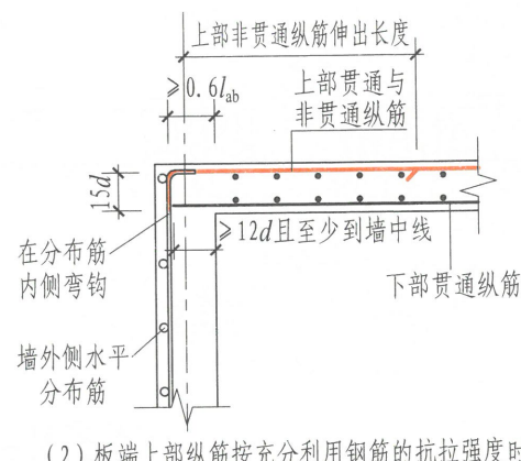
(2) 板端上部纵筋按充分利用钢筋的抗拉强度时
