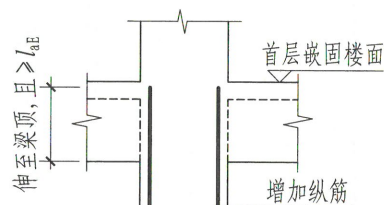
(b) 直锚
