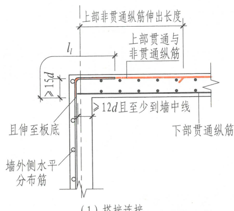
(1) 搭接连接
