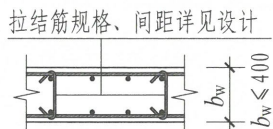
剪力墙双排配筋
