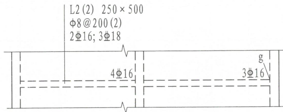
图4.2.4-5 梁一端采用充分利用钢筋抗拉强度方式的注写示意 注:“g”表示右端支座按照非框架梁Lg配筋构造。
