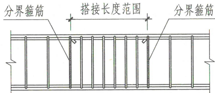
梁、柱类构件纵向受力钢筋搭接接头区箍筋构造
