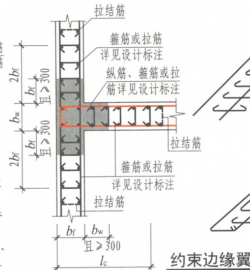
约束边缘翼墙 (一)
