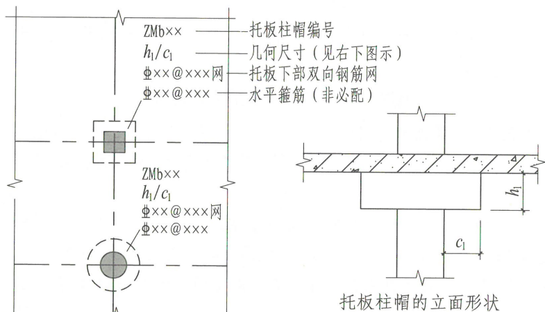
图7.2.3-2 托板柱帽ZMb引注图示
