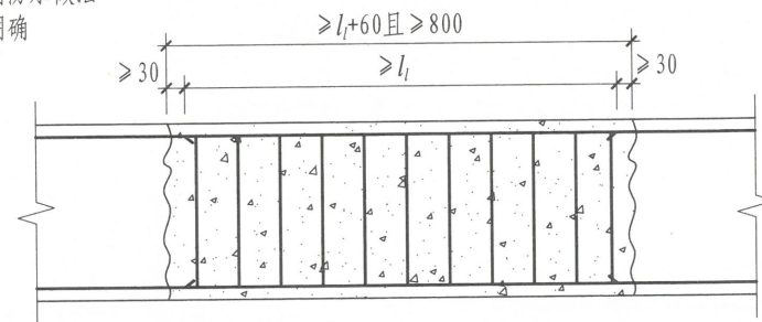
梁后浇带HJD100%搭接钢筋构造
