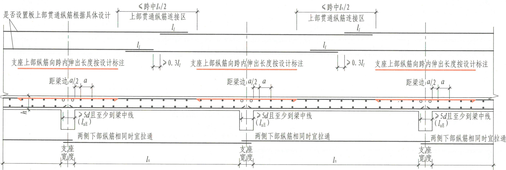
有梁楼盖楼面板LB和屋面板WB钢筋构造
