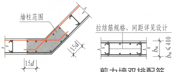
斜交转角墙
