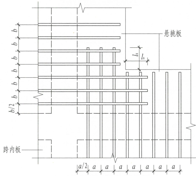
悬挑板阴角构造 (一) (本图未表示构造筋及分布筋)
