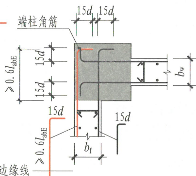
端柱转角墙 (二)
