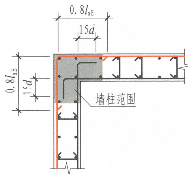
转角墙 (三)
