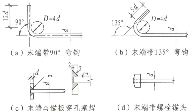
纵向钢筋弯钩与机械锚固形式
