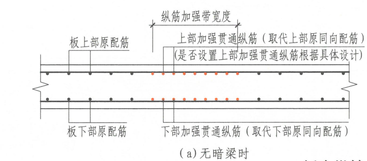
板内纵筋加强带JQD构造 (加强贯通纵筋的连接要求与板纵筋相同)
