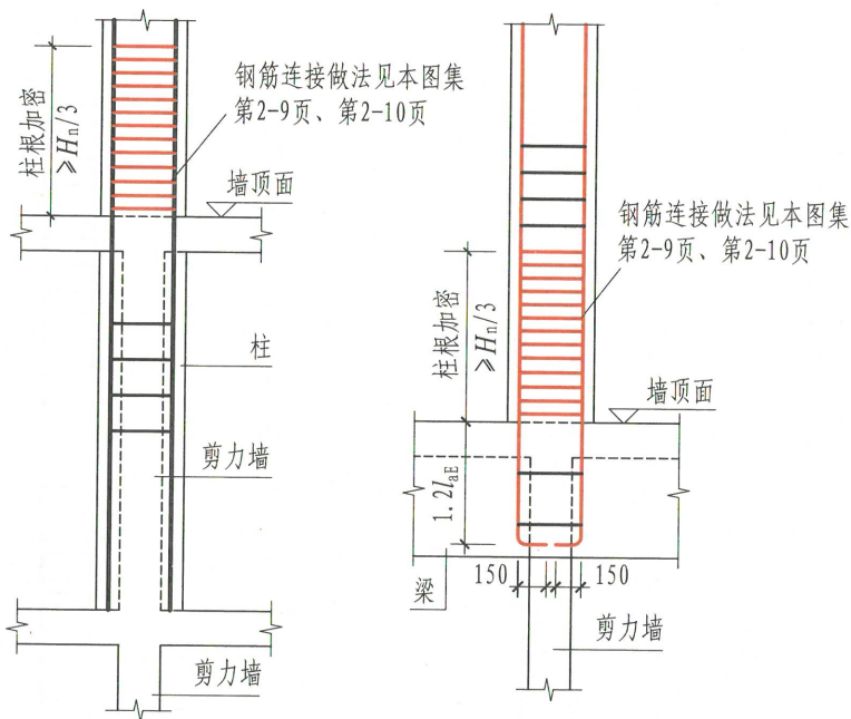
(b) 柱纵筋锚固在墙顶部时柱根构造
