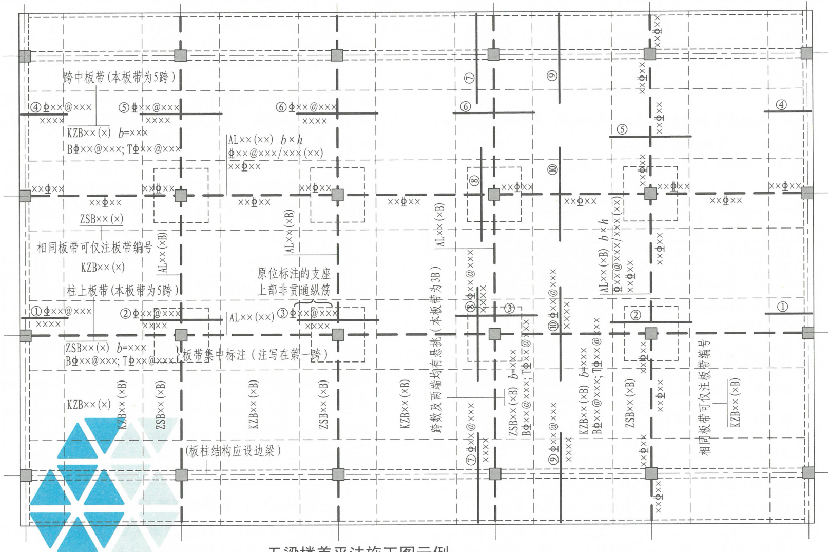
无梁楼盖平法施工图示例 (板厚均为xxx)
