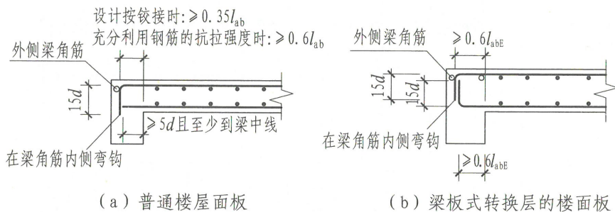
板在端部支座的锚固构造 (一)
