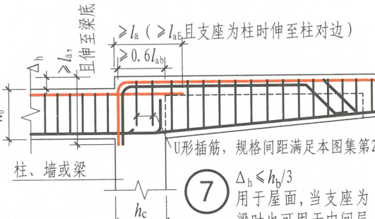
⑥ \Delta_h \leq h_b/3 用于屋面，当支座为梁时也可用于中间层
