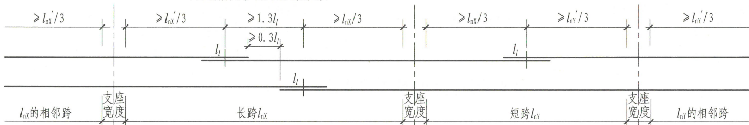
(B) 不等跨板上部贯通纵筋连接构造(二)
