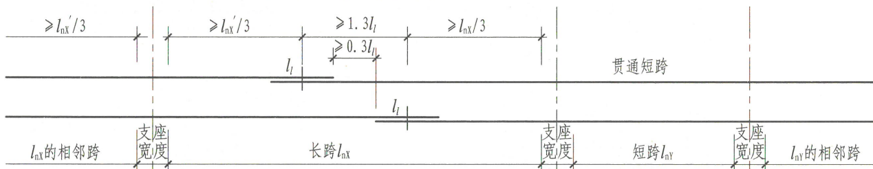
(C) 不等跨板上部贯通纵筋连接构造(三)
