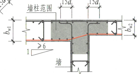
翼墙 (三)
