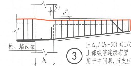
② \Delta_h / (h_c - 50) > 1/6 仅用于中间层
