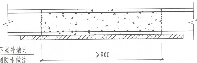
墙后浇带HJD钢筋贯通构造
