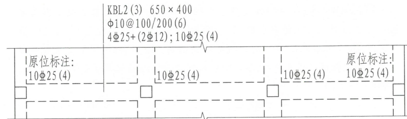
图4.2.5 框架扁梁平面注写方式示例
