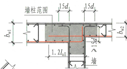
翼墙 (二)
