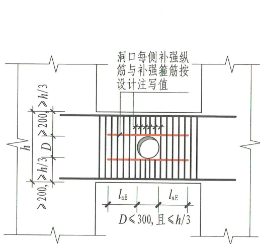
连梁中部圆形洞口补强钢筋构造 (圆形洞口预埋钢套管)
