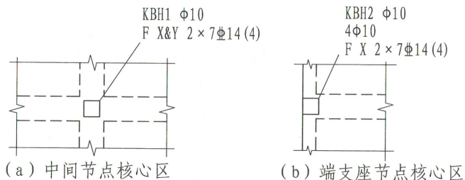
图4.2.6 框架扁梁节点核心区附加钢筋注写示意图、施工时应注意:
