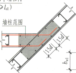
斜交翼墙
