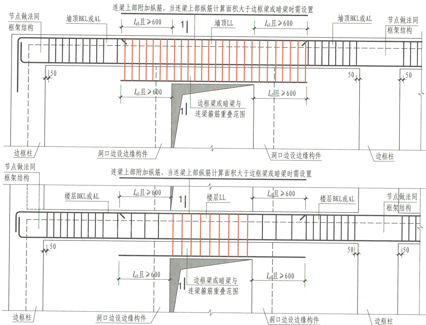
剪力墙BKL或AL与LL重叠时配筋构造
