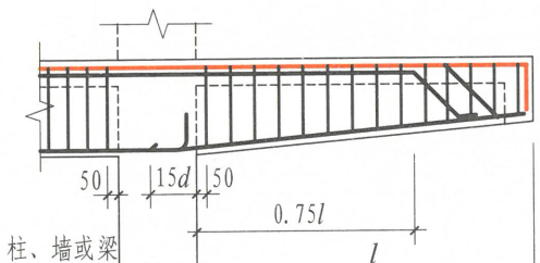
① 可用于中间层或屋面
