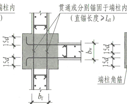
端柱翼墙 (二)
