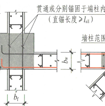
端柱翼墙 (三)
