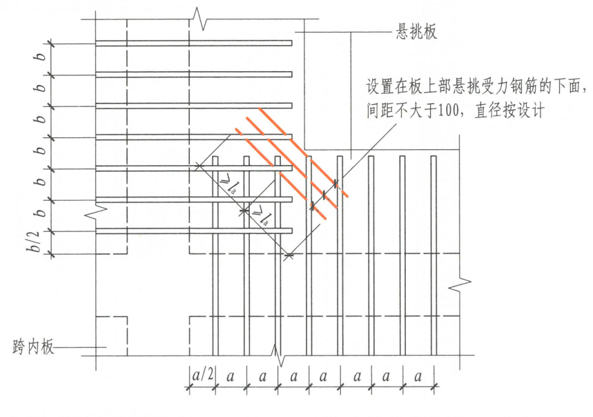
悬挑板阴角构造 (二)
