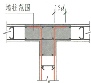
翼墙 (一)
