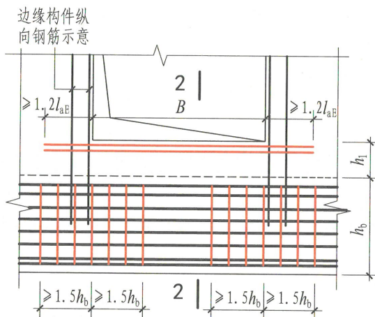
( B > 2h_1 且 h_1 < h_0/2 )
