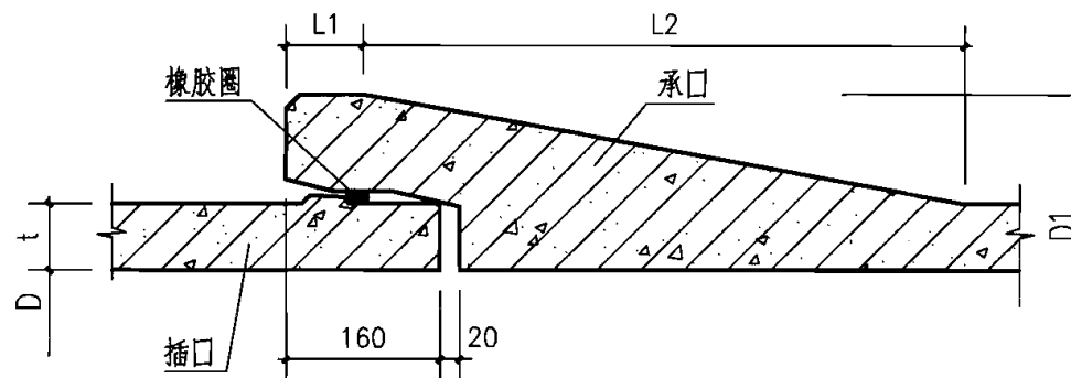
接口大样
