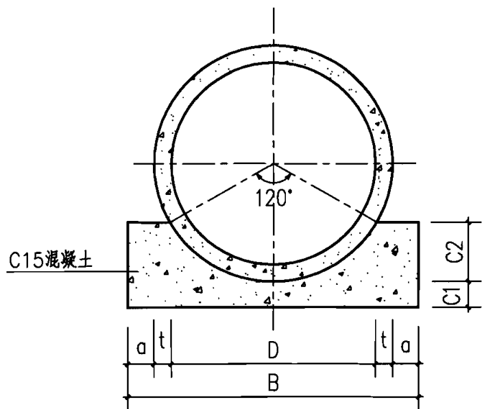
基础断面图
