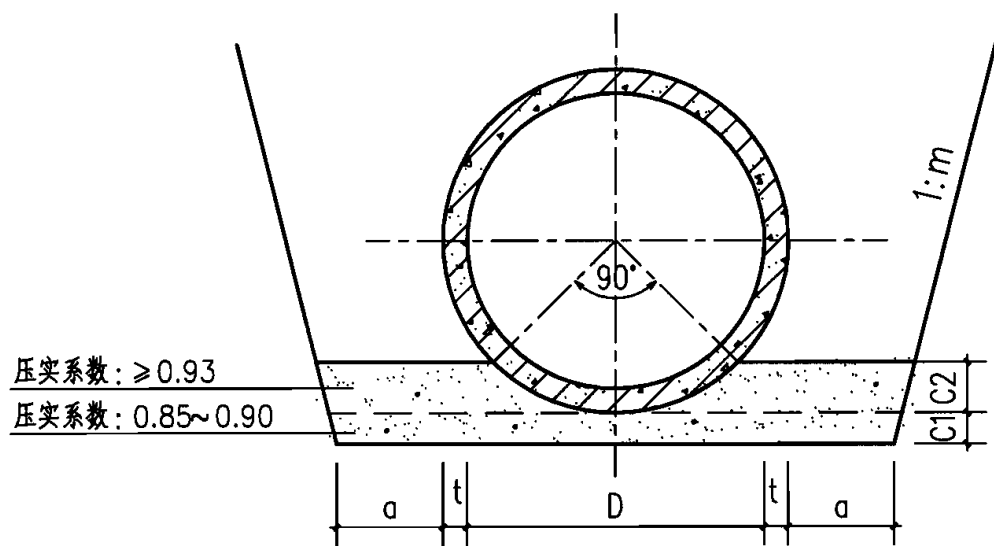
基础断面图
