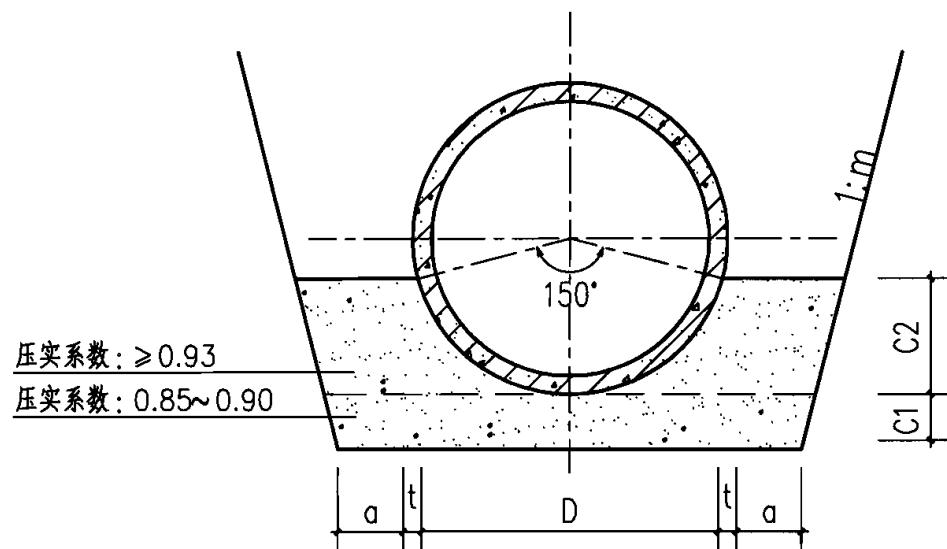
基础断面图
