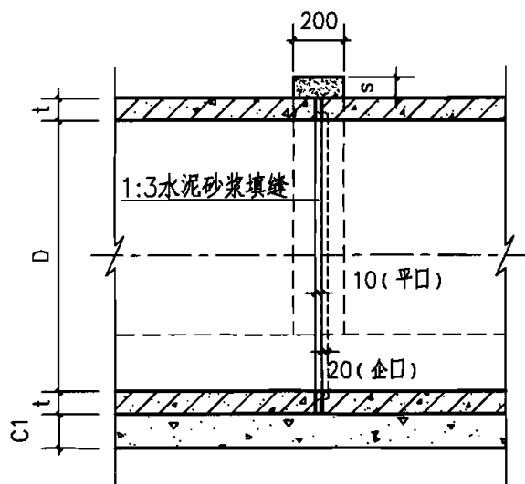
接口纵断面
