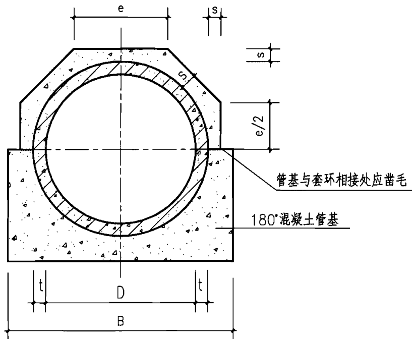
接口横断面
