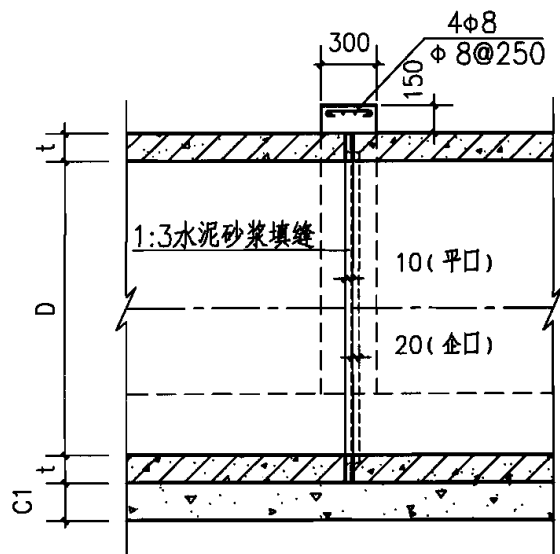
接口纵断面
