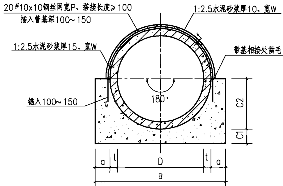
接口横断面
