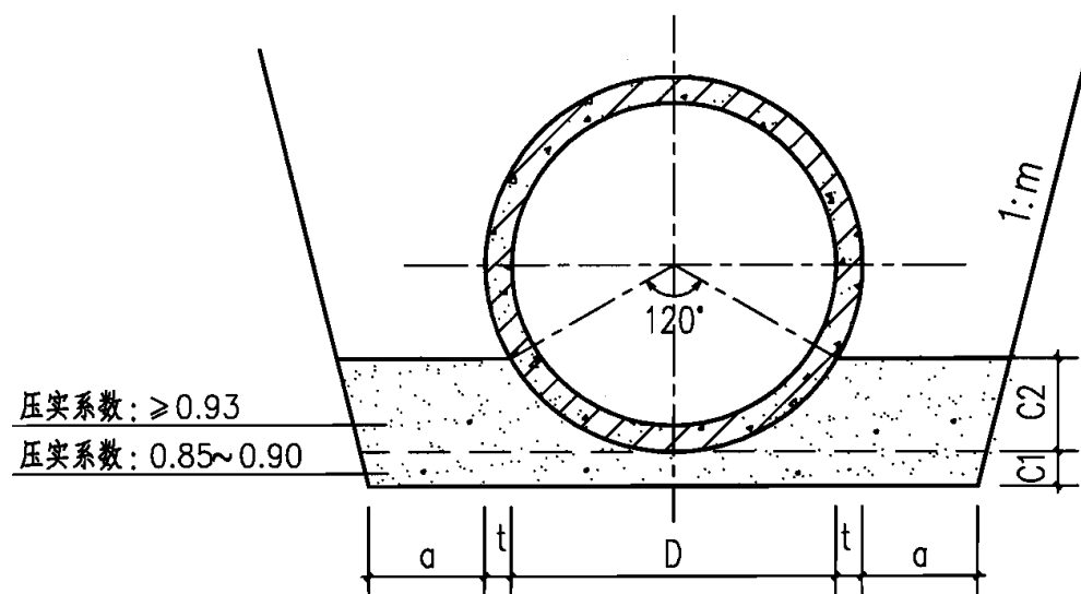
基础断面图
