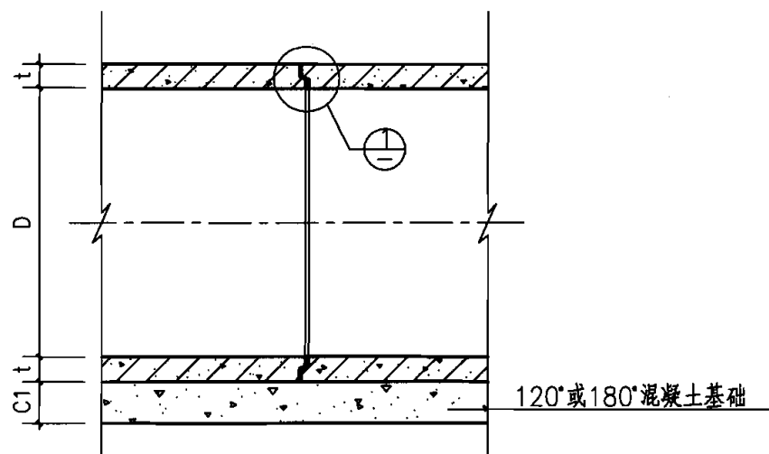
接口纵断面
