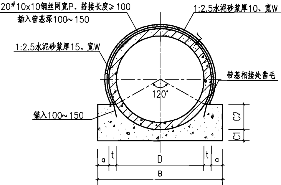
接口横断面
