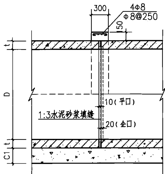
接口纵断面
