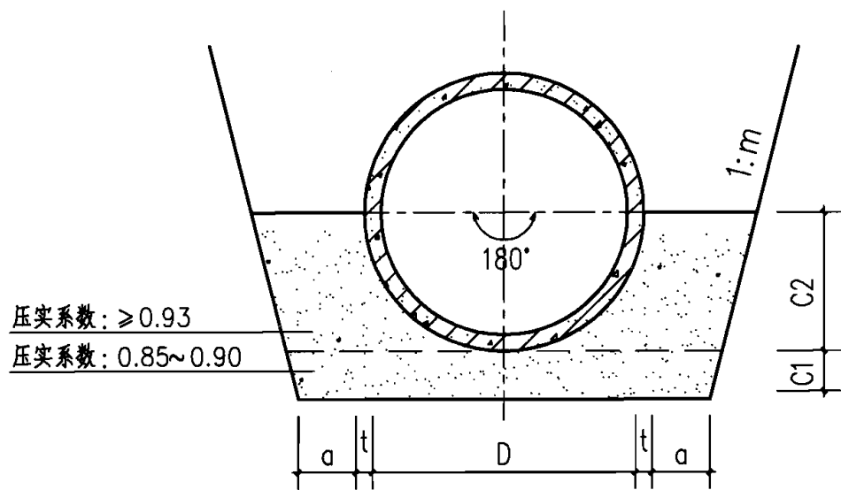
基础断面图
