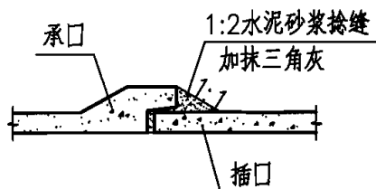
承插口管接口示意图
