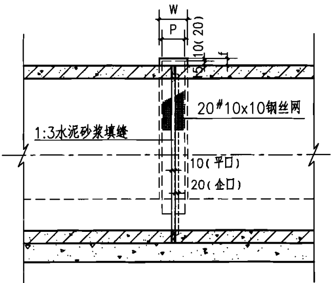
接口纵断面
