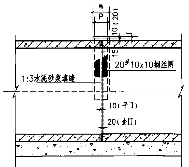
接口纵断面
