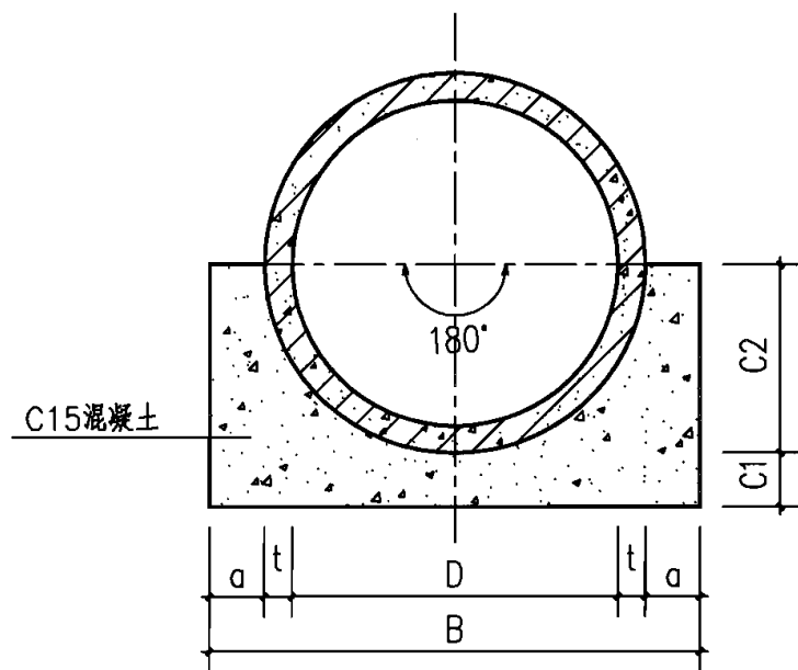
基础断面图
