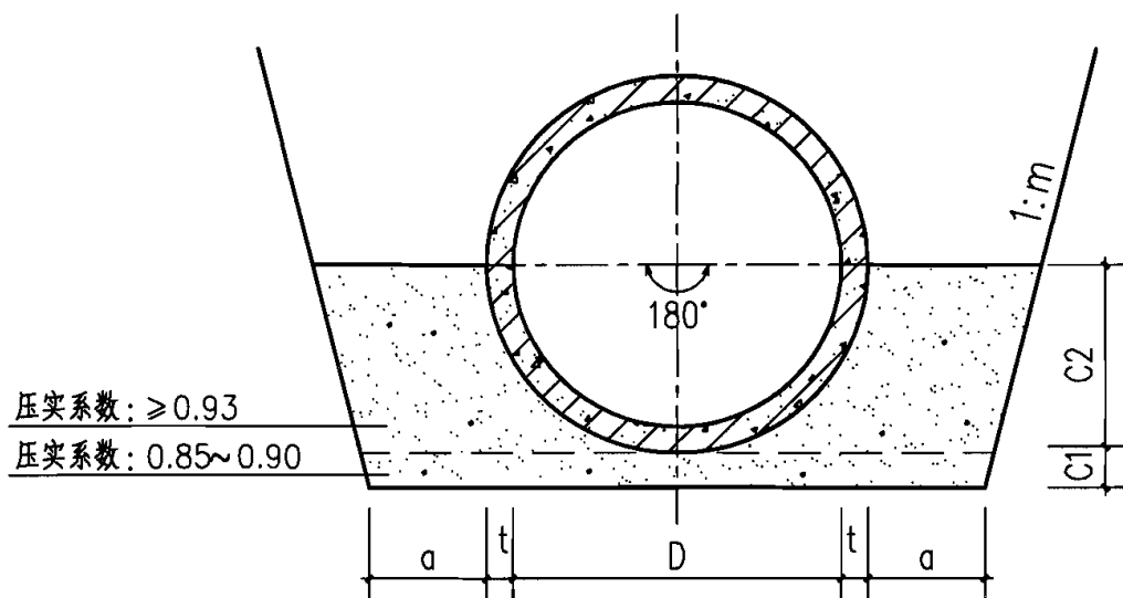
基础断面图
