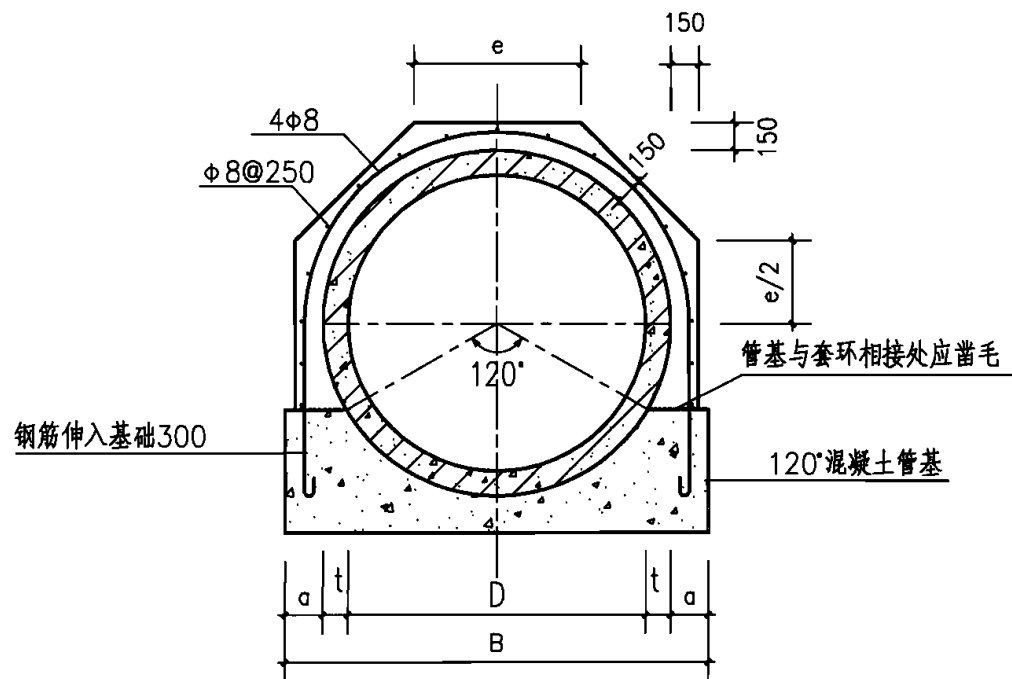
接口横断面
