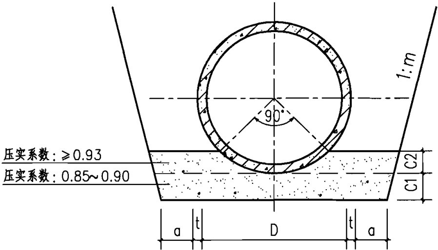
基础断面图
