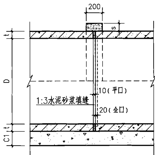
接口纵断面
