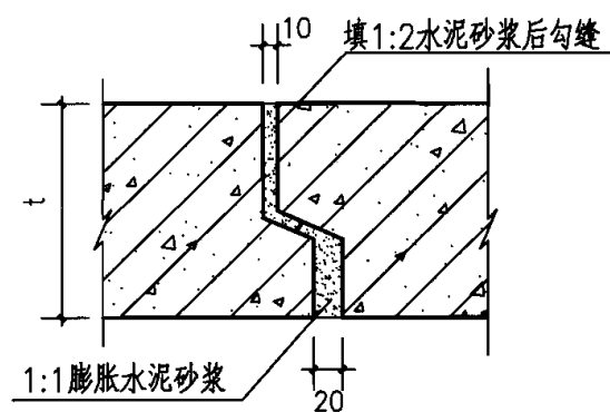
① 接口大样
