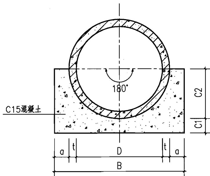
基础断面图
