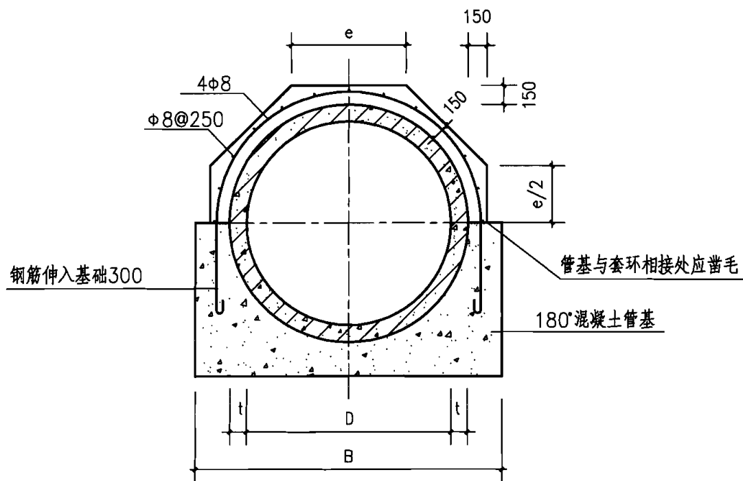
接口横断面
