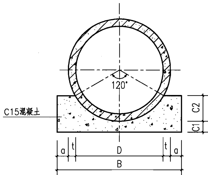
基础断面图
