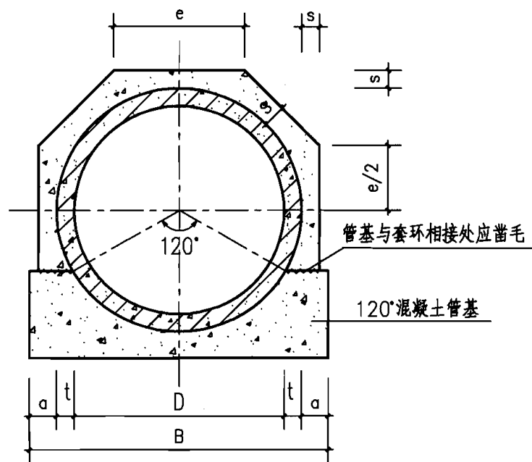
接口横断面
