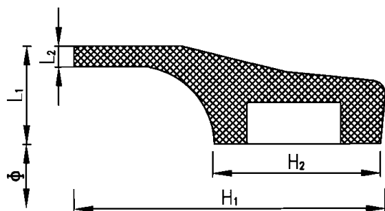
橡胶圈截面
