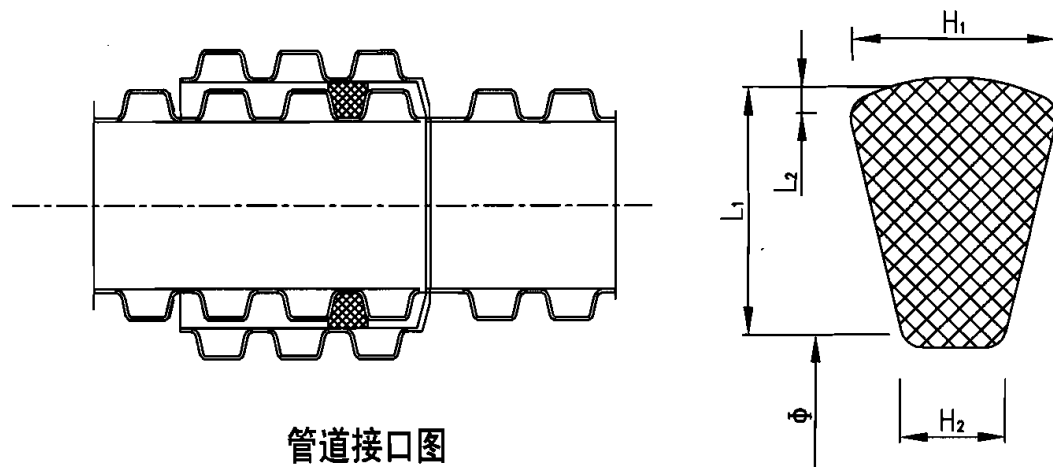
橡胶圈截面图
