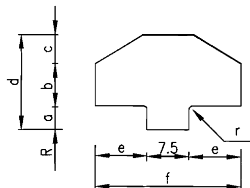
橡胶圈截面图
