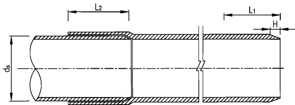
胶粘剂接口
