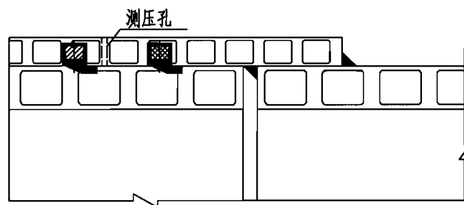
污水承插式接口
