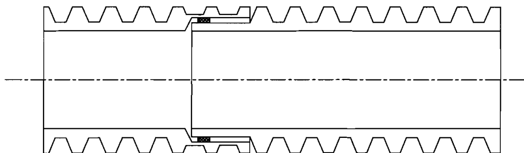
管道接口图
