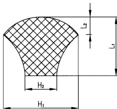
De400~De800橡胶圈截面
