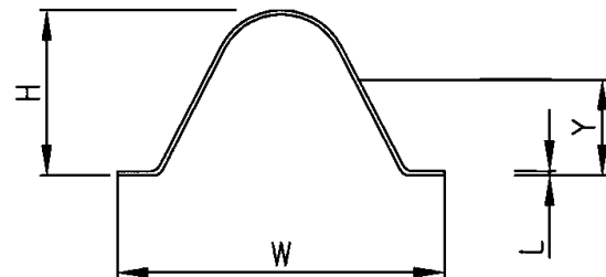
U2型截面示意图
