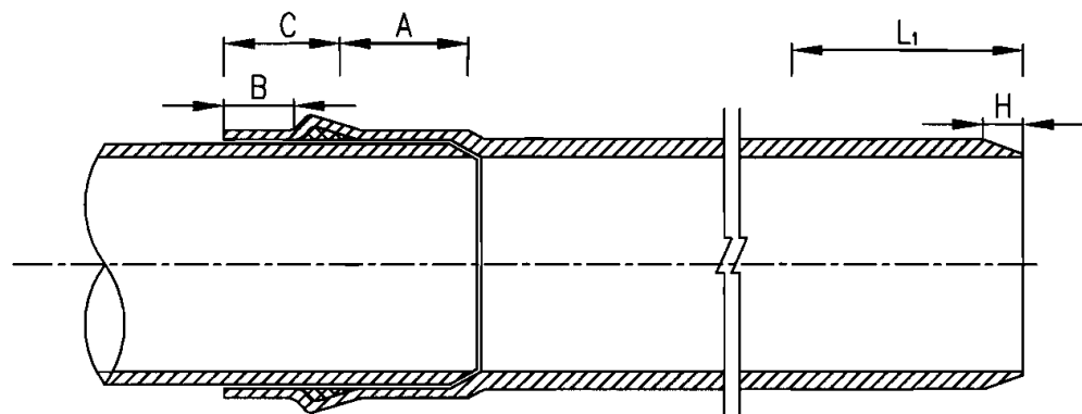
橡胶圈接口
