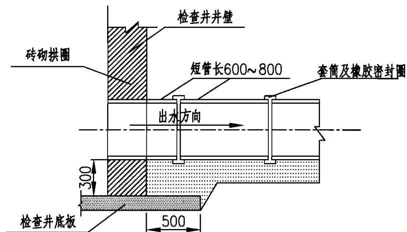
落底检查井
