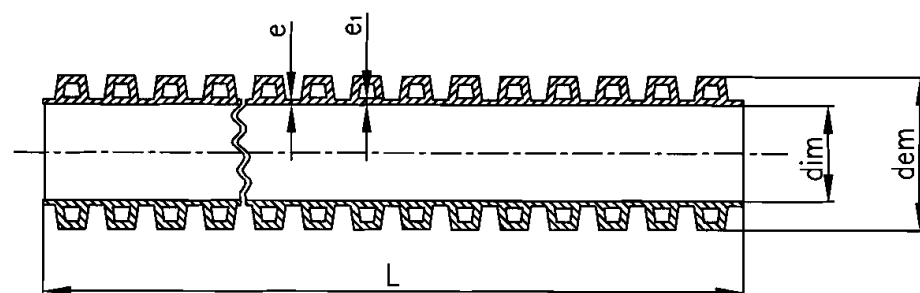
不带扩口管材结构示意图
