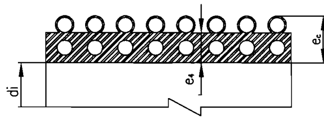
B型结构壁管的典型示例2
