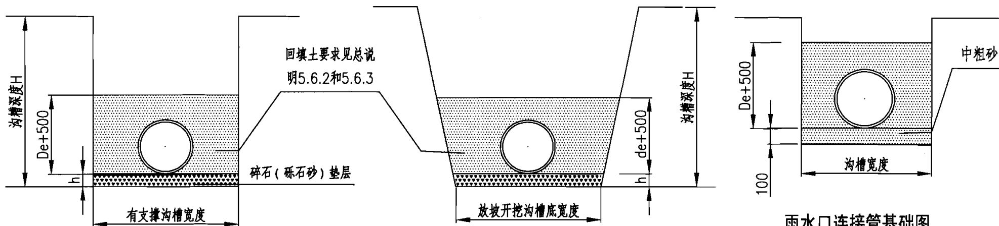
雨水口连接管基础图
