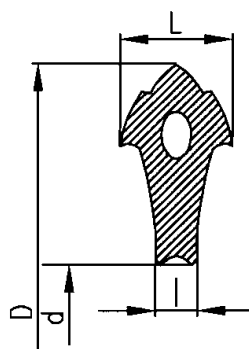
密封圈截面
