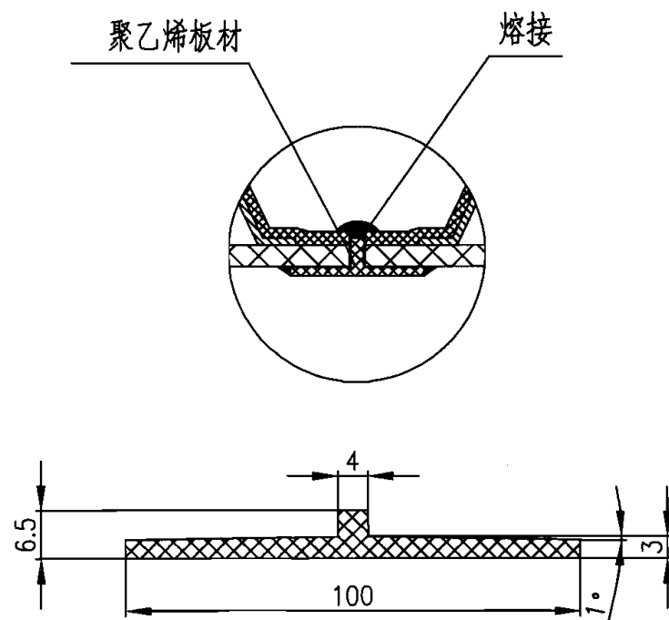
聚乙烯板材尺寸
