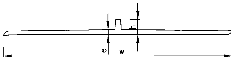
PVC-U钢塑复合缠绕管接口示意图
