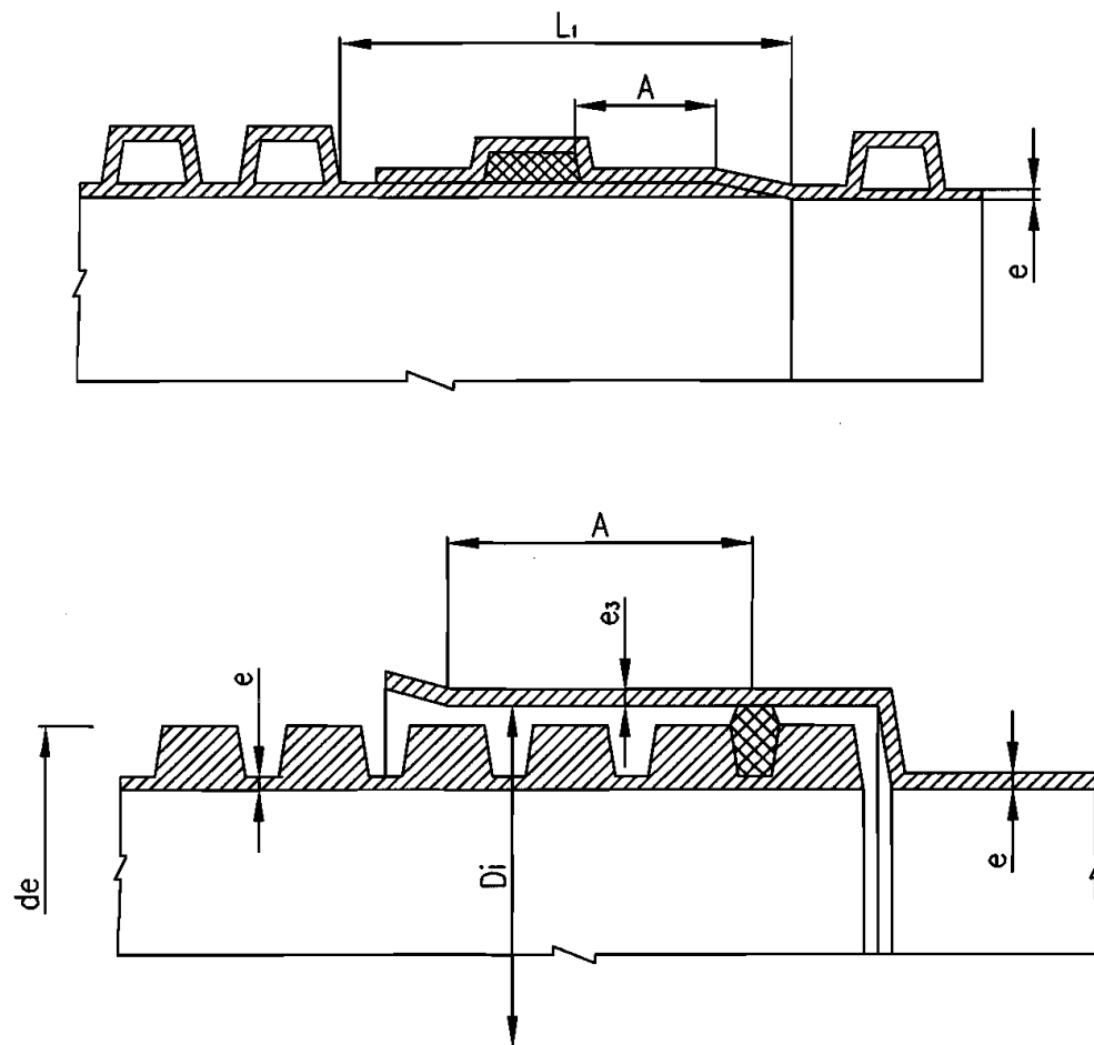
管材承插口
